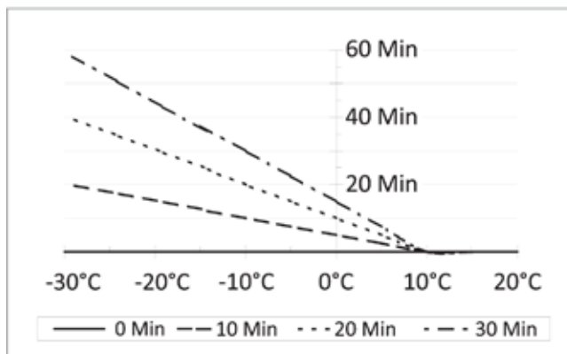
Abb. 24: Vorhaltezeit
