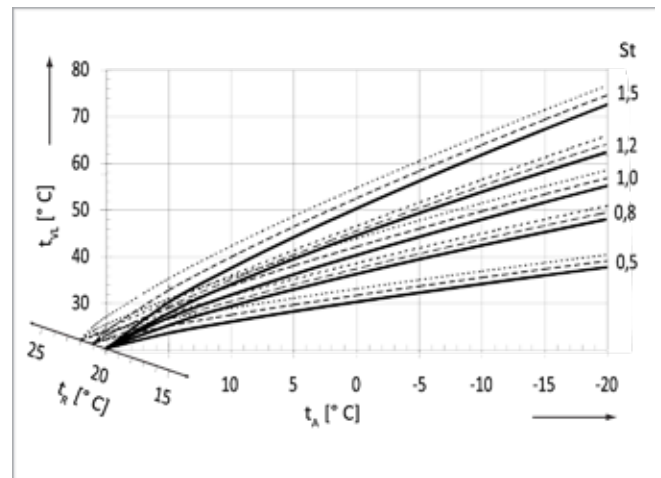
Abb. 23: Heizkurven bei diversen Raumsolltemperaturen
