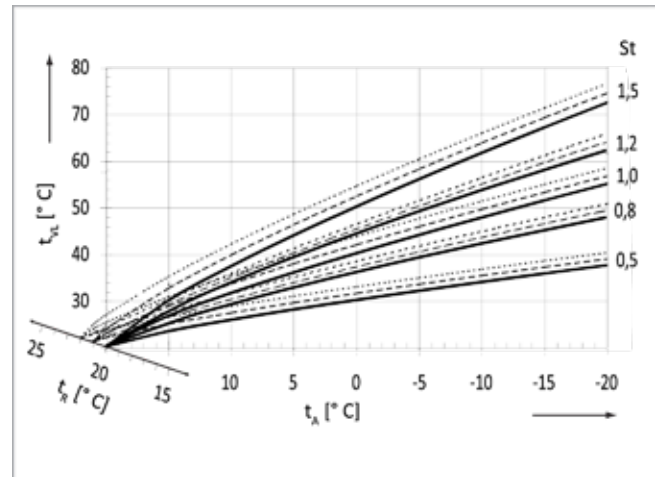
Abb. 26: Heizkurven bei diversen Raumsolltemperaturen
